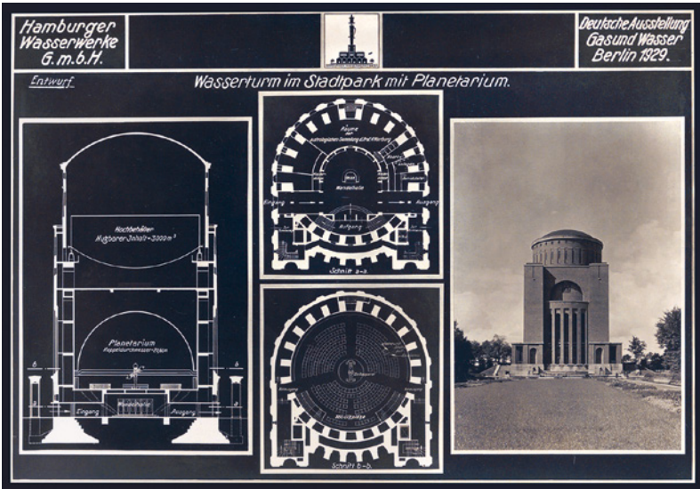
Abbildung 9: Postkarte mit Entwurf des Hamburger Planetariums im Wasserturm. Hamburg 1929. Quelle: Staatsarchiv Hamburg.
