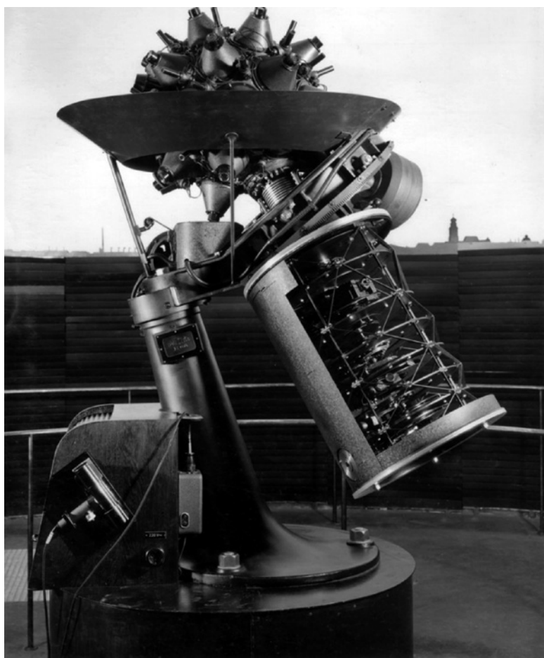
Abbildung 14: Planetariumsprojektor Model I mit Lichtzeiger im Deutschen Museum. München 1925. Quelle: Deutsches Museum, München.
