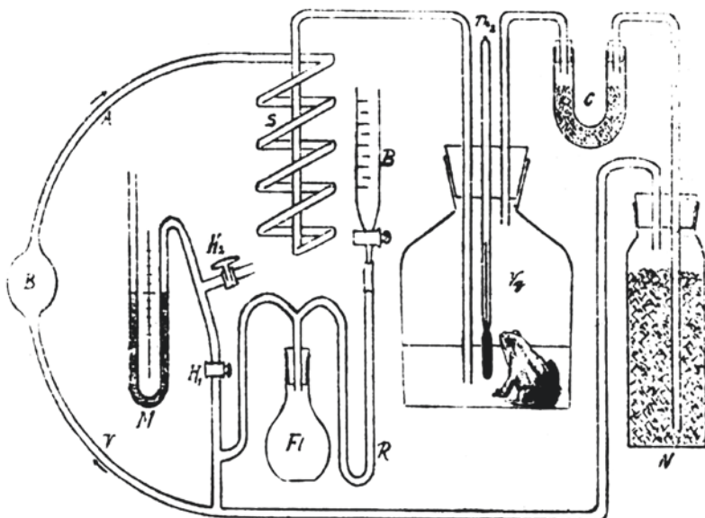
Abb. 1: Respiroapparat nach Cohnheim, modifiziert von Joel (1919)
