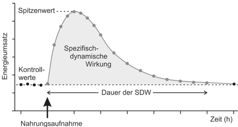
Abb. 2: Schematische Darstellung der Steigerung des Sauerstoffverbrauchs bzw. des Energieumsatzes nach Nahrungsaufnahme. Der Umsatz erreicht einen Spitzenwert nach etwa einer Stunde, die gesamte spezifisch-dynamische Wirkung entspricht der grau markierten Fläche unter der Kurve.
